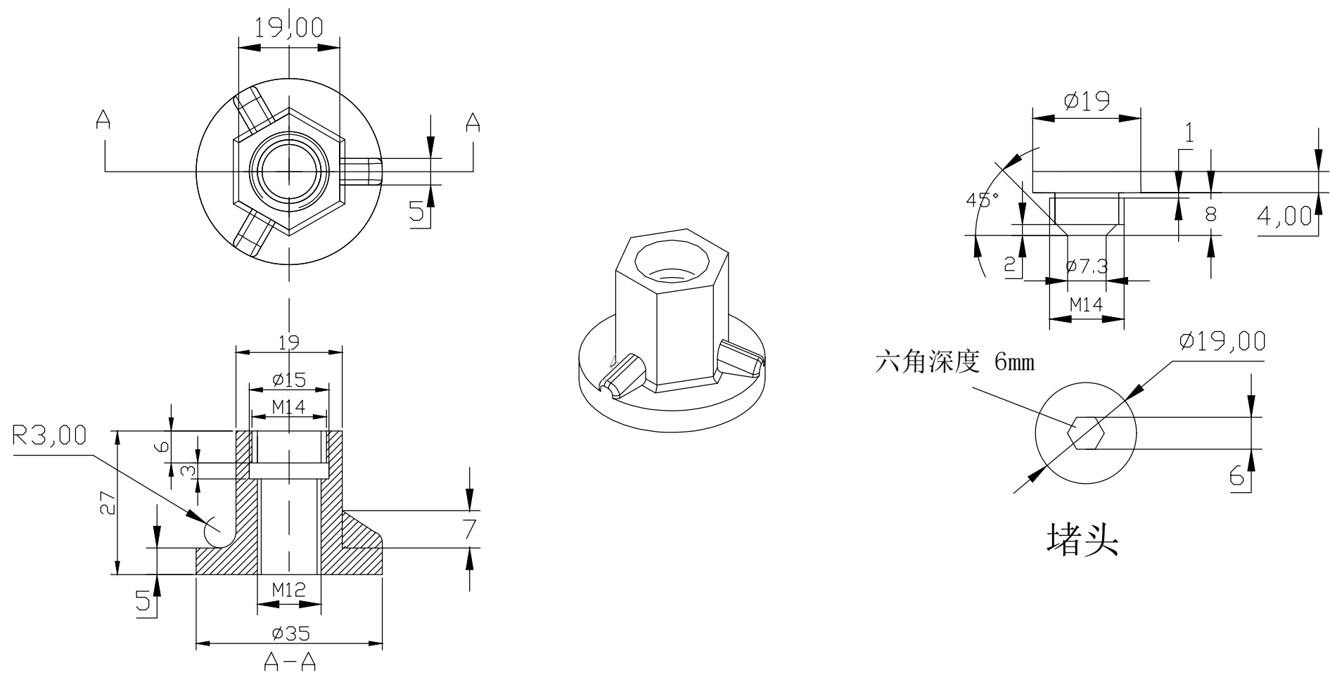
预埋构件大样图
